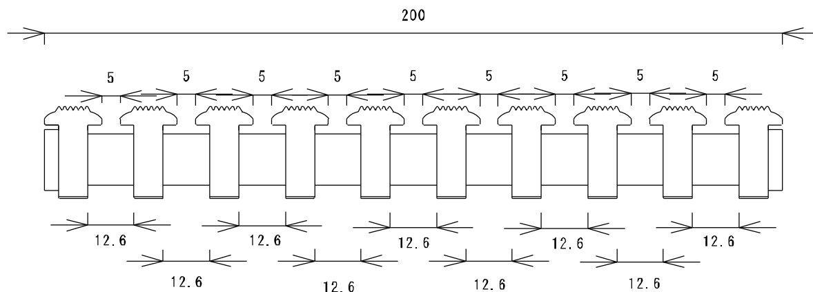
断面図 A-A スケール 1 : 1
